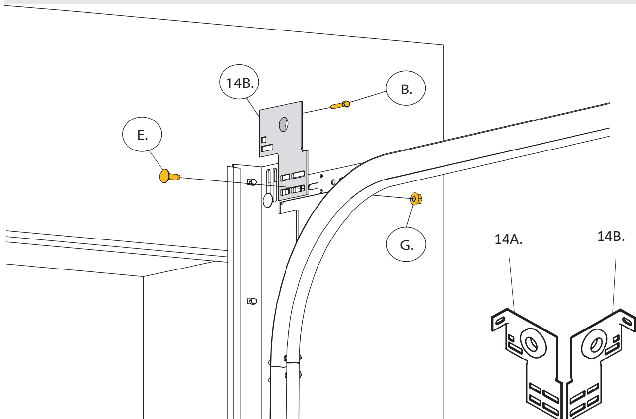
Figur 8 - Montering av endebraketter.
